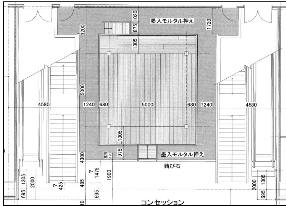
江戸舞台平面図
